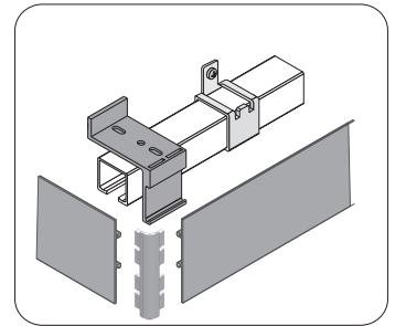
Díszléc és saroktoldó a K-075-ös sínhez
