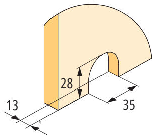
az alsó görgő nyílása
