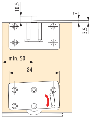
a görgők elhelyezése és méretei
