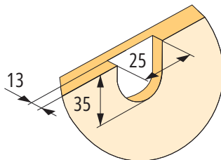
a felső görgő nyílása
