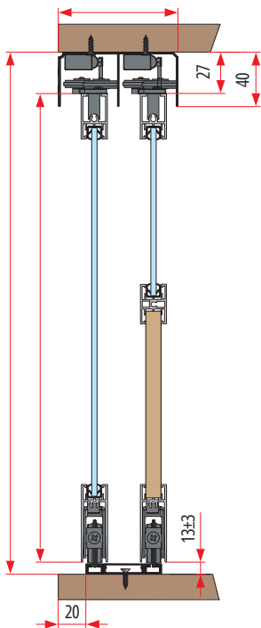
Rapid sîn csillapítóval
