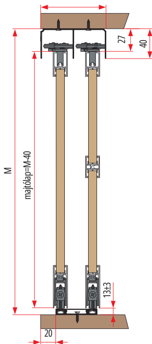
Rapid sîn pozícionálóval
